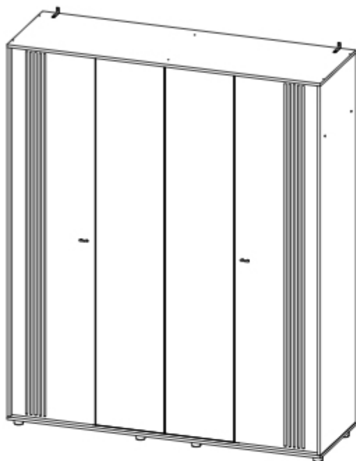
Модульная система «Милан» Шкаф четырехстворчатый 1801x2200x561 (ШxВxГ)
