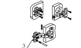
Регулировка створки по высоте
