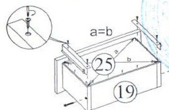
Порядок сборки выдвижного ящика
