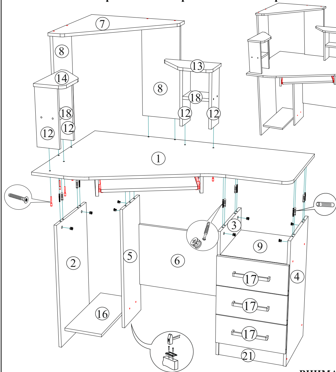
Рис.3 - Схема сборки Компьютерный стол «Каспер»
