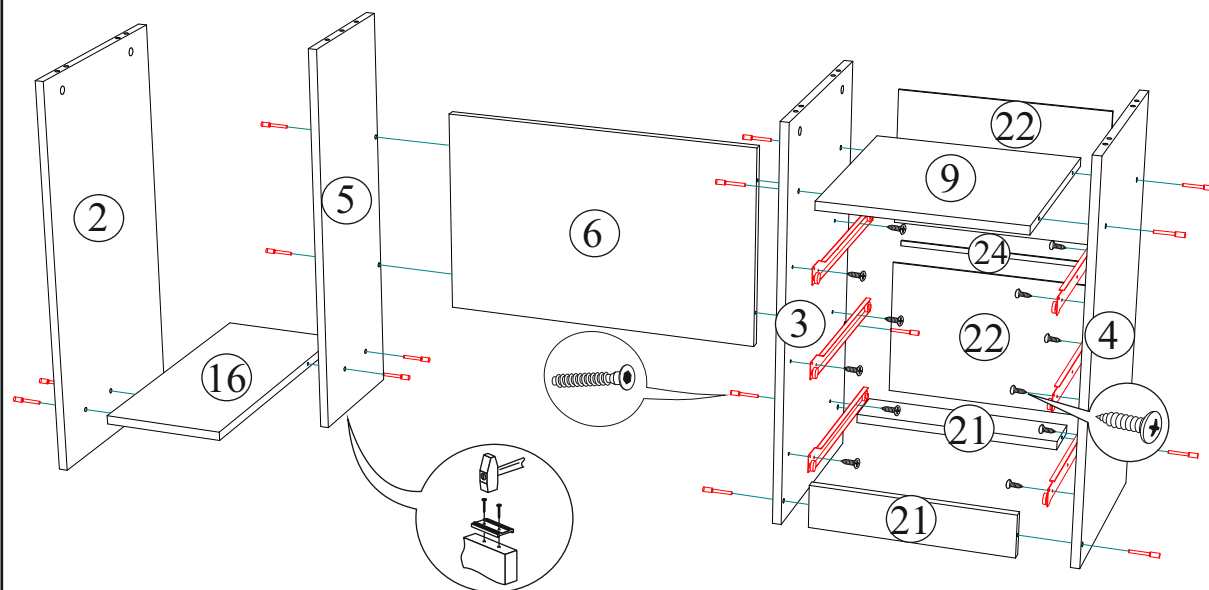
рис.2 Рис.2 - Схема сборки нижней части Компьютерный стол «Каспер»
