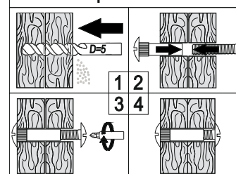
Схема установки межсекционной стяжки
