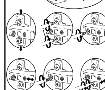
Установка и регулировка петель
