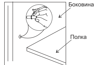
Установка полкодержателя.
