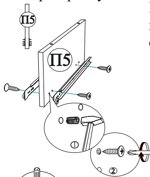
Рис.2 Прикручивание направляющих на перегородку П5
