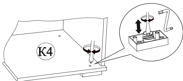
Рис.8 Регулировка опор
