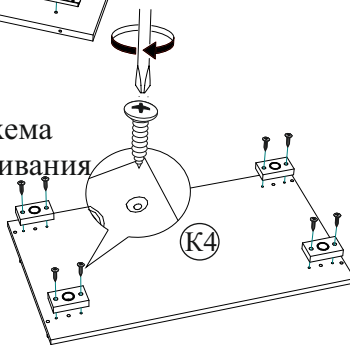
Рис.4 Схема расстановки шкантов и эксцентриковых стяжек
