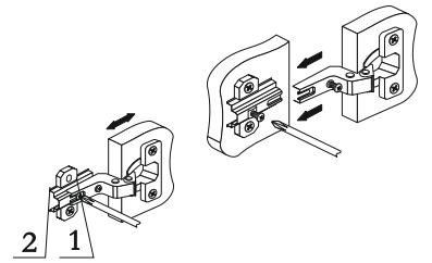
Регулировка створки по ширине
