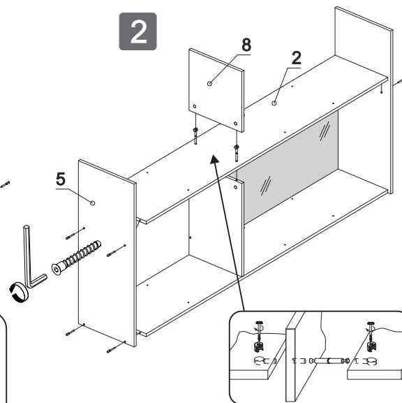
Установка двухсторонней эксцентриковой стяжки
