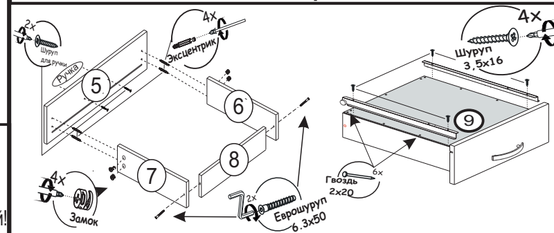
Схема сборки ящика
