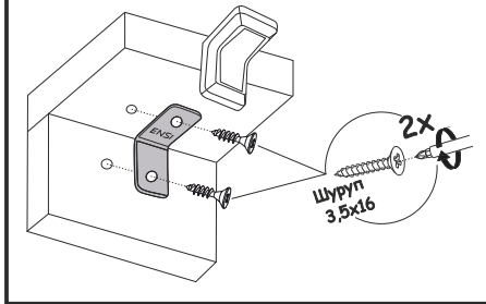
Схема установки уголка с накладкой
