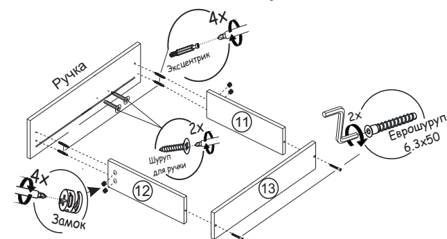
Рис.7 Схема сборки ящика
