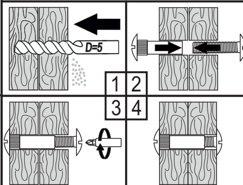
Схема установки межсекционной стяжки
