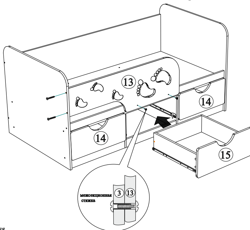
Рис.5 Установка декора и ящика
