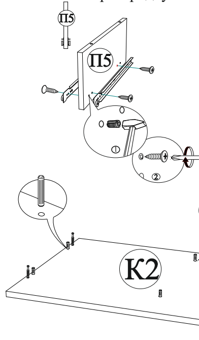
Рис.2 Прикручивание направляющих на перегородку П5
